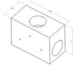
HPPA-00-00T9 Standard 9/16" Tee
